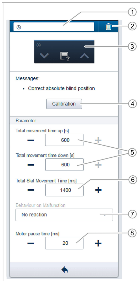
Fig. 54: Actuator settings
